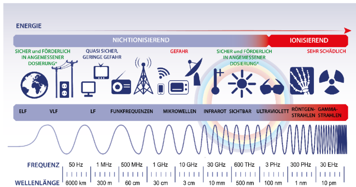
Abbildung 1 – Elektromagnetisches Spektrum
